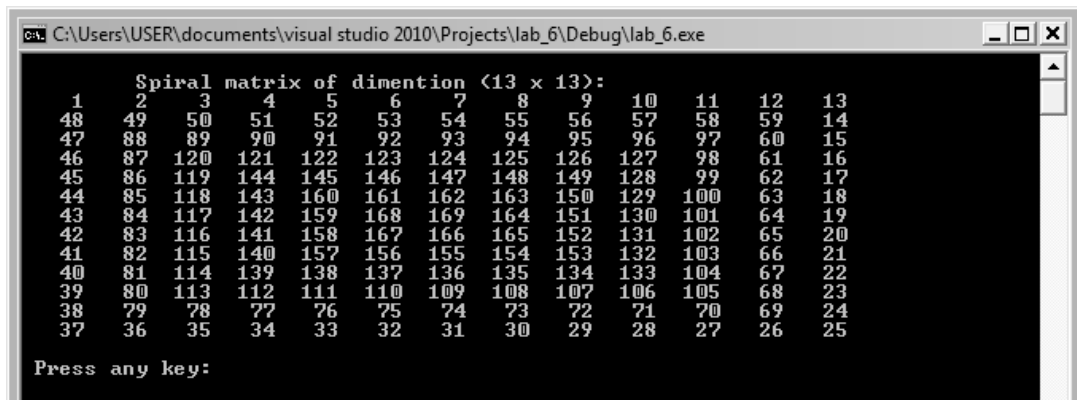
Рисунок 6.2 – Заполнение матрицы по спирали
