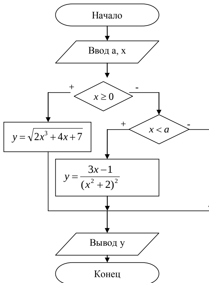
Рисунок 3.7 – Блок-схема к заданию
