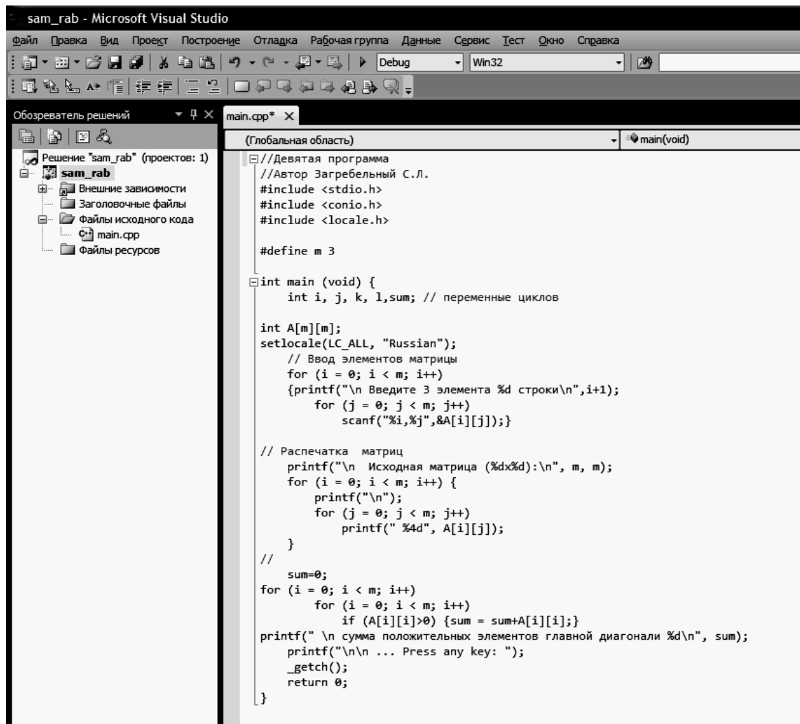
Рисунок 9.2 – Окно кода программы
