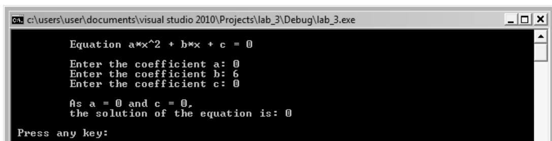
Рисунок 3.2 – Выполнение программы с двумя нулевыми коэффициентами
