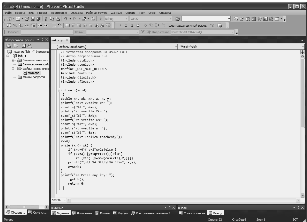
Рисунок 4.7 – Окно программы
