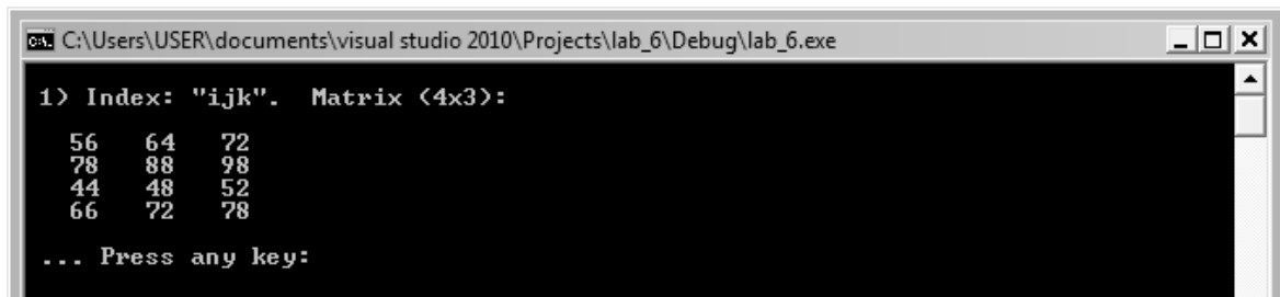
Рисунок 6.4 – Результат произведения двух матриц
