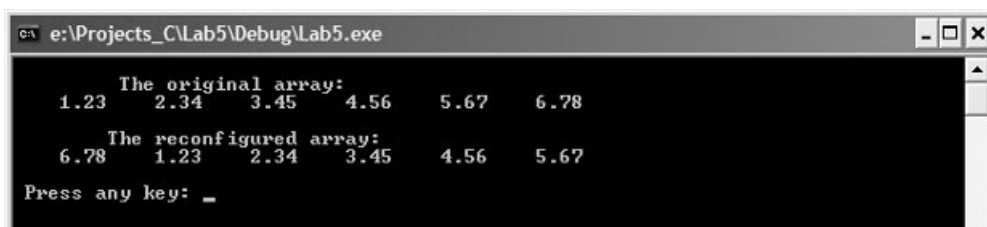
Рисунок 5.3 – Пример циклической перестановки элементов числового массива
