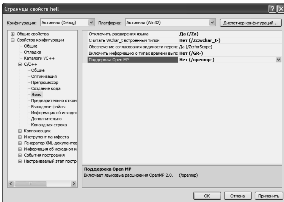
Рисунок 1.15 – Страница свойств закладки Язык
