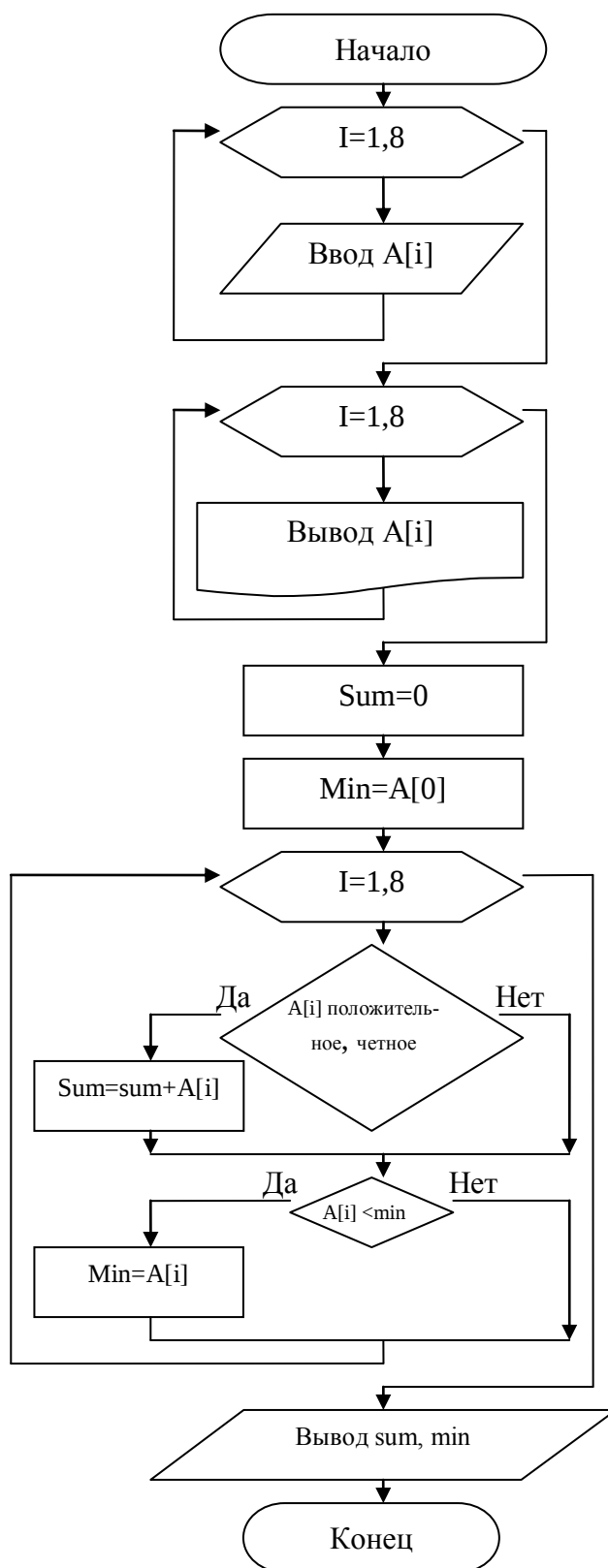
Рисунок 5.5 – Блок-схема к заданию
