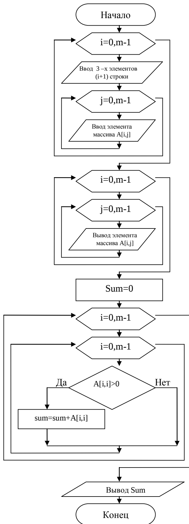
Рисунок 9.1 – Блок-схема к программе
