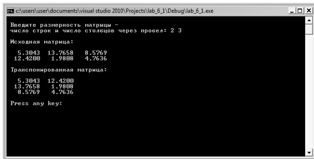
Рисунок 6.5 – Пример транспонирования матрицы
