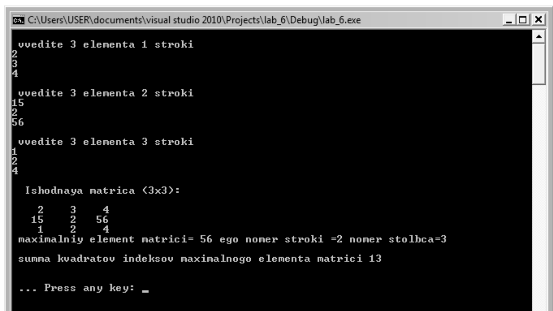
Рисунок 6.8 – Обработка элементов матрицы
