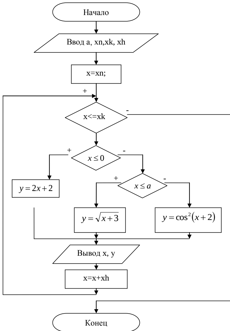
Рисунок 4.6 – Блок-схема к заданию
