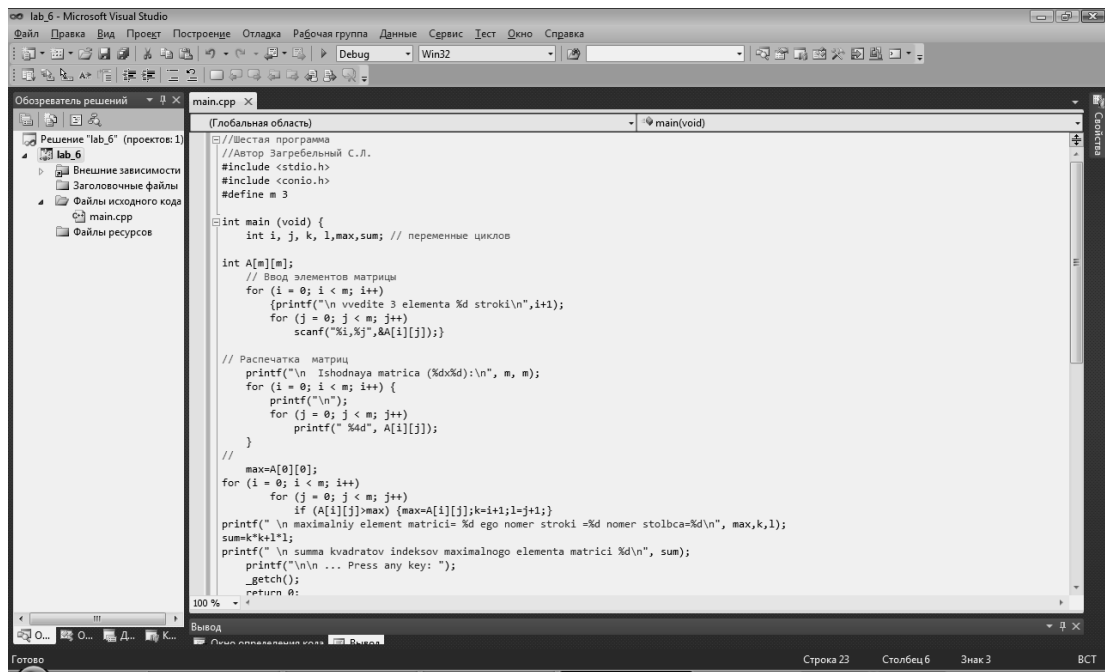
Рисунок 6.7 – Окно примера
