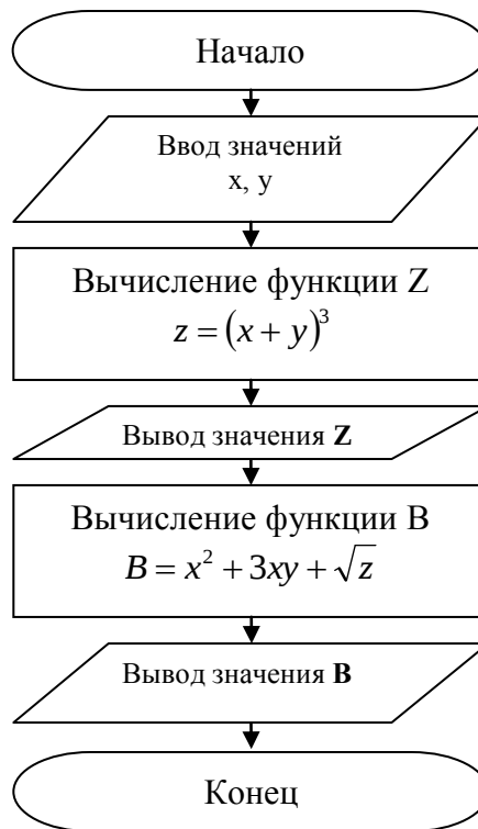
Рисунок 2.3 – Блок-схема примера 2
