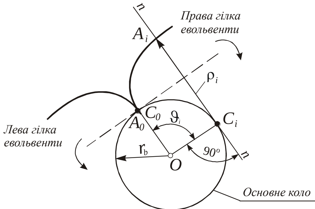
Рисунок 1 – Евольвента кола
