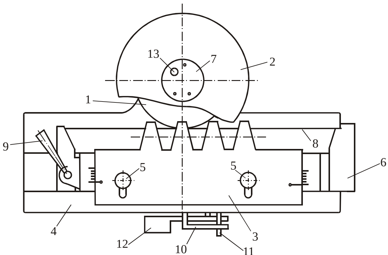
Рисунок 8 – Схема приладу ТММ-42
