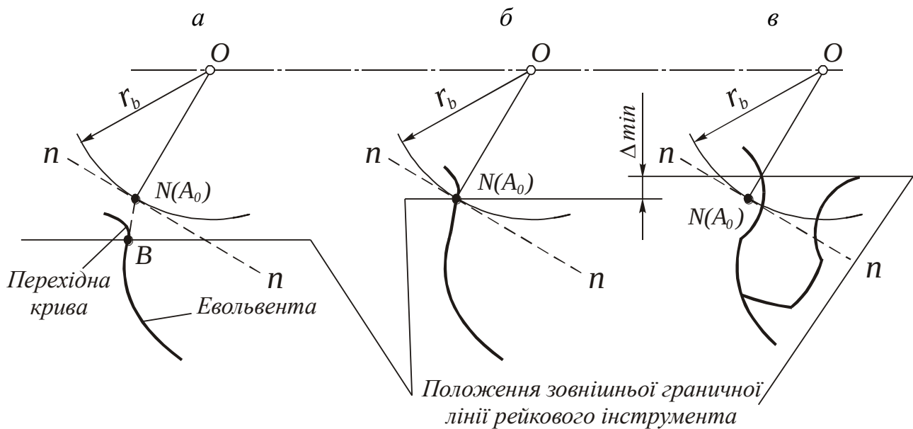
Рисунок 7 – Можливі варіанти нарізання нульових евольвентних зубчастих коліс
