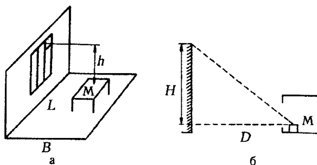
Рисунок 5.3 – Естественное боковое освещение помещения
