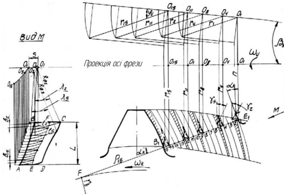
Рисунок 2.1 – Графічний спосіб побудування кконтактного поля різання правого корпусу черв'ячної фрези з роздільною схемою формоутворення
