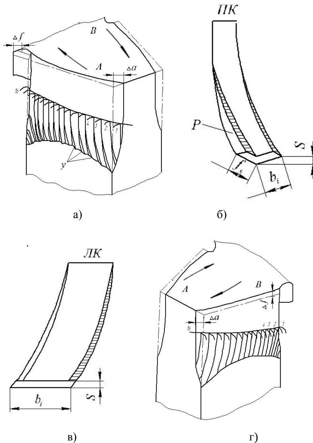
Рисунок 2.3 – Форма шарів, різаних зубами правозахідної фрези з роздільною схемою формоутворення: а - утворення уступів (Y) при роботі правого корпусу; б - форма шару, різаного зубами правого корпусу; в - форма шару, різаного зубами лівого корпусу; г - схема обробки поверхні зуба лівим корпусом
