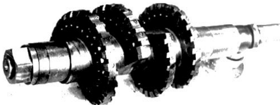
Рисунок 4.6 - Чистова черв'ячна фреза з роздільною схемою формоутворення m = 12 мм у зборі з оправкою
