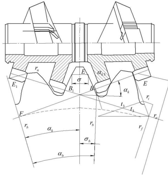
Рисунок 3.8. – Схема верстатного зачеплення спеціальної твердосплавної фрези з оброблюваним колесом
