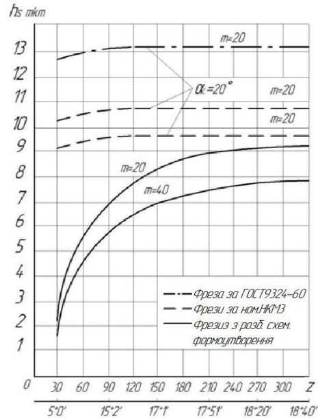
Рисунок 3.2 – Залежність максимальної розрахункової висоти хвилі від кількості зубів нарізованого колеса для фрез різних виконань
