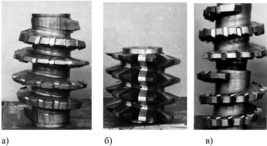
Рисунок 4.1 – Експериментальний зубофрезерний інструмент : а – черв'ячна фреза з роздільною схемою формоутворення m = 20\text{мм} ; б – стандартна черв'ячна фреза m = 20\text{ мм} (ГОСТ 9324 -60); в) - черв'ячна фреза з роздільною схемою формоутворення m = 28\text{ мм}
