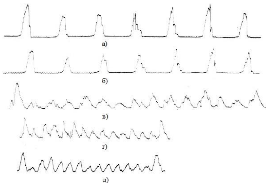
Рисунок 4.2 – Характерні осцилограми крутних моментів при чистовому нарізуванні колеса m = 20\text{мм} ; z = 96 ; а- стандартна фреза S = 4\text{мм/об} , V = 16\text{м/хв} (зустрічне фрезерування з обробкою дна западин зубів); б- без обробки дна западин зубів; в - черв'ячна фреза з роздільною схемою формоутворення S = 4\text{мм/об} ; 16\text{м/хв} , зустрічне фрезерування; г - фреза з роздільною схемою формоутворення S = 4\text{мм/об} , V = 30\text{м/хв} , зустрічне фрезерування; д - попутне фрезерування
