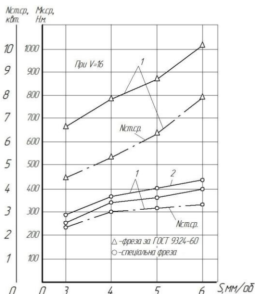
Рисунок 4.3 – Залежність середнього крутного моменту M_{к.сер} та середньої споживаної верстатом потужності N_{ст.сер} від подачі черв'ячних фрез S при оброблюванні колеса m = 20 м q 20 мм; z = 95 ; 1-зустрічне фрезерування; 2 - попутне фрезерування
