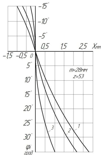
Рисунок 2.5 – Відхилення проєкцій траєкторій точок різальних кромek від площини профілювання в залежності від кута повороту фрези.
