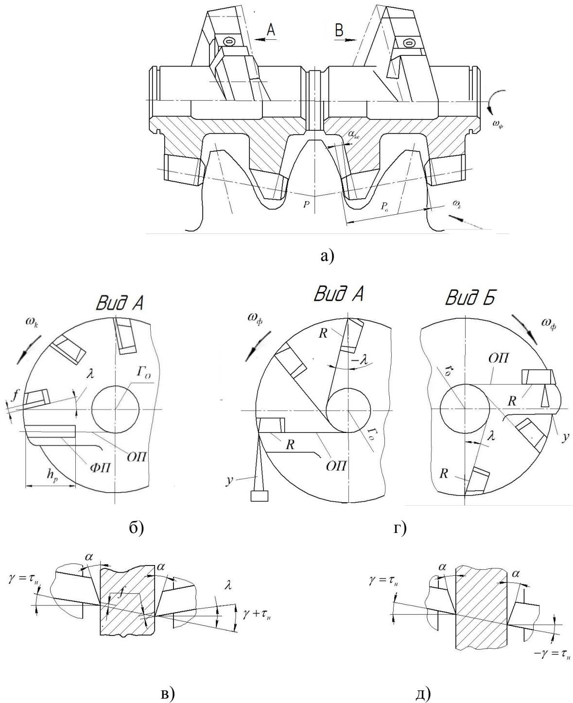
Рисунок 3.7 – Профілювання черв'ячних фрез із роздільною схемою формоутворення на основі евольвентного черв'яка: а - схема оброблення зубів колеса корпусами фрези; б - розташування зубів фрези з гвинтовою стрічкою; в - геометрія різальної частини фрези за наявності гвинтової стрічки; г - розташування зубів фрези в площинах, дотичних до основного циліндра; д - геометрія різальної частини фрези без гвинтової стрічки
