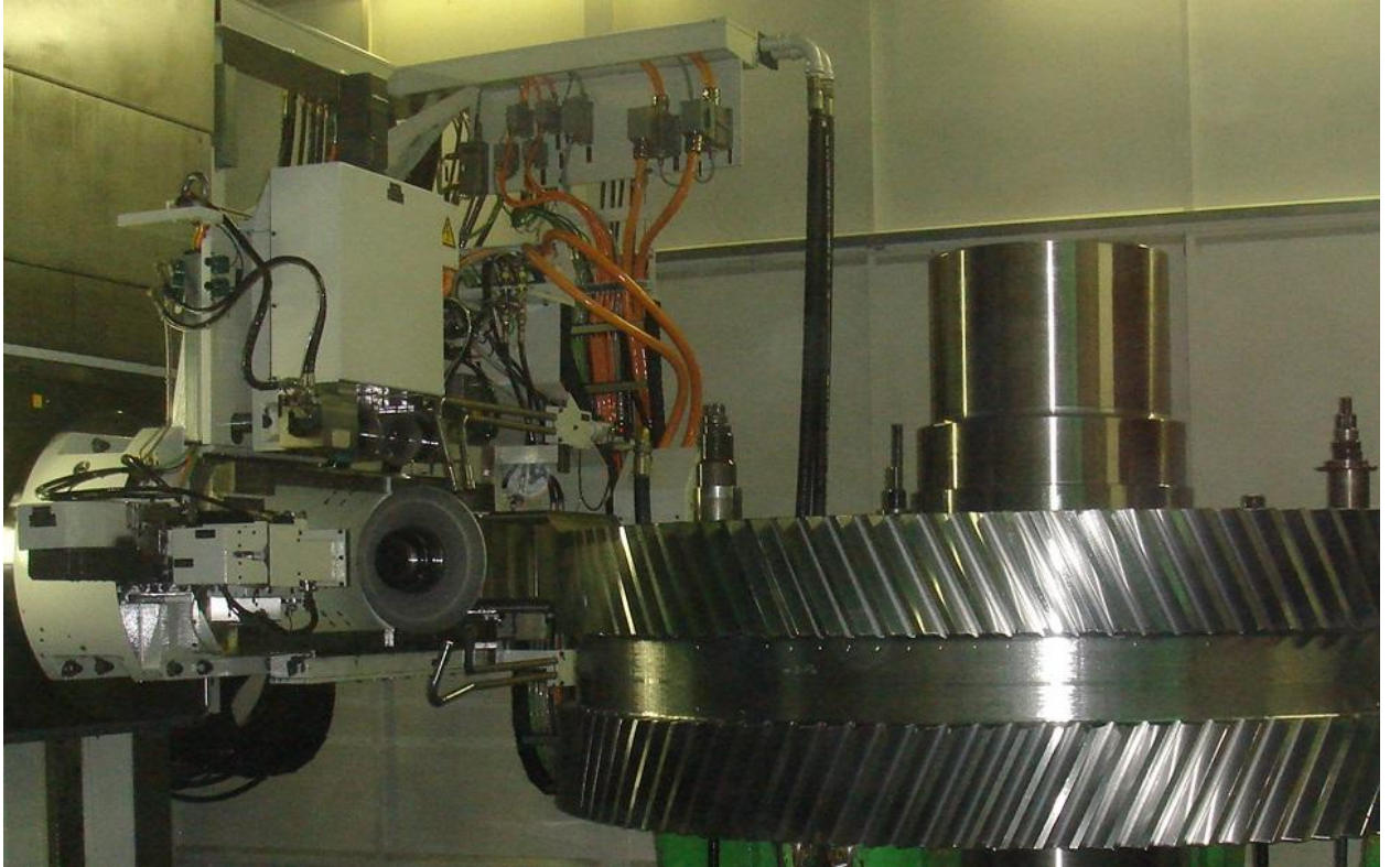
Рисунок 1.3 – Зубофрезерування шевронних коліс на верстаті з ЧПУ
