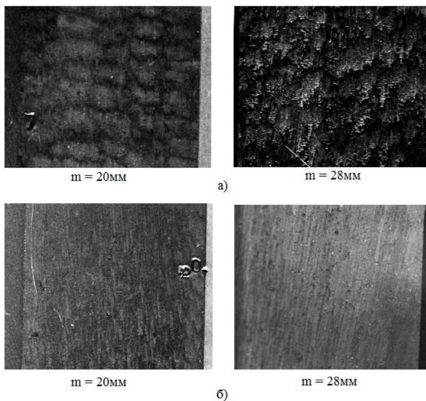
Рисунок 5.3 - Вид бічної поверхні зубів коліс m = 20\text{мм} и m = 28\text{мм} (\Delta = 0,5\text{м}; S = 4 \text{ мм/об}; V = 16 \text{ м/хв}) : а - оброблення стандартною фрезою; б оброблення фрезою з роздільною схемою формоутворення
