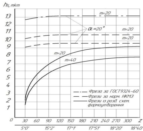
Рис. 7 – Залежність максимальної розрахункової висоти хвилі від кількості зубів нарізуваного колеса для фрез різних виконань
