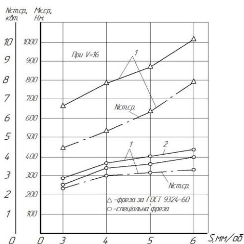
Рис. 13 – Залежність середнього крутного моменту M_{к.ср} та середньої споживаної верстатом потужності N_{ст.ср} від подачі черв'ячних фрез S при оброблюванні колеса m = 20\text{ мм} , z = 95 : 1-зустрічне фрезерування; 2 - попутне фрезерування
