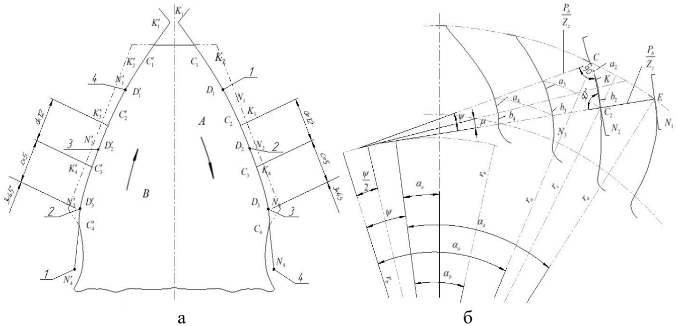
Рис. 1 – Визначення ширини зрізуваних шарів:
