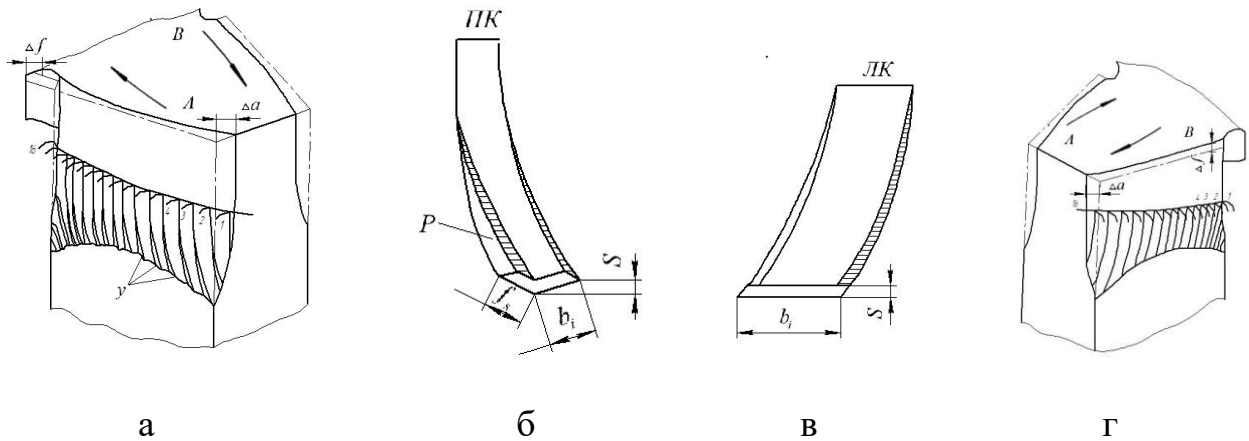
Рис. 2 – Форма шарів, зрізуваних зубами правозахідної фрези з роздільною схемою формоутворення: а - утворення уступів (У) при роботі правого корпусу; б - форма шару, зрізуваного зубами правого корпусу; в - форма шару, зрізуваного зубами лівого корпусу; г - схема обробки поверхні зуба лівим корпусом
