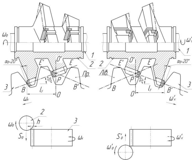
Рис. 10 – Схема оброблення зубів колеса одним правим корпусом фрези: а), с) – правий корпус при зустрічному фрезеруванні; б), д) - правий корпус при попутному фрезеруванні
