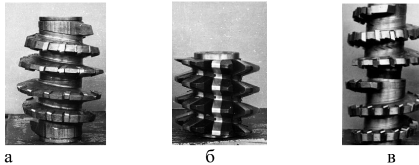
Рис. 12 - Експериментальний зубофрезерний інструмент:
