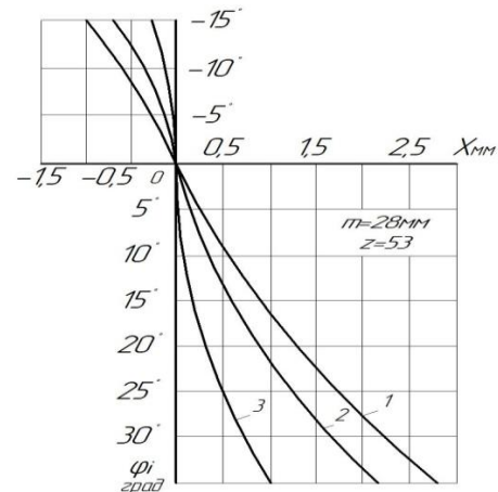
Рис. 4 – Відхилення проекцій траєкторій точок різальних кромок від площини профілювання у залежності від кута повороту фрези. Зони обробки: 1 - вершина зубного колеса; 2 - дільний діаметр; 3 - основа зуба
