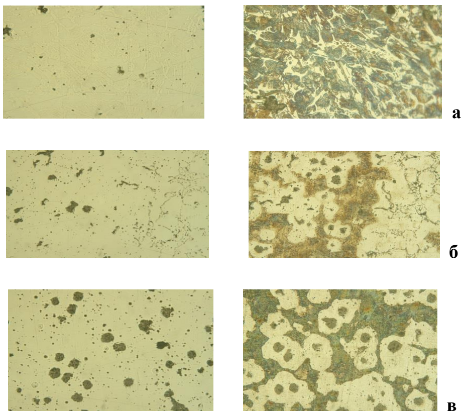
Рисунок 5 - Микроструктура чугуна в поверхностной зоне (а), в зоне сплавления двух порций (б) и в центральной зоне отливки «Цилиндр»
