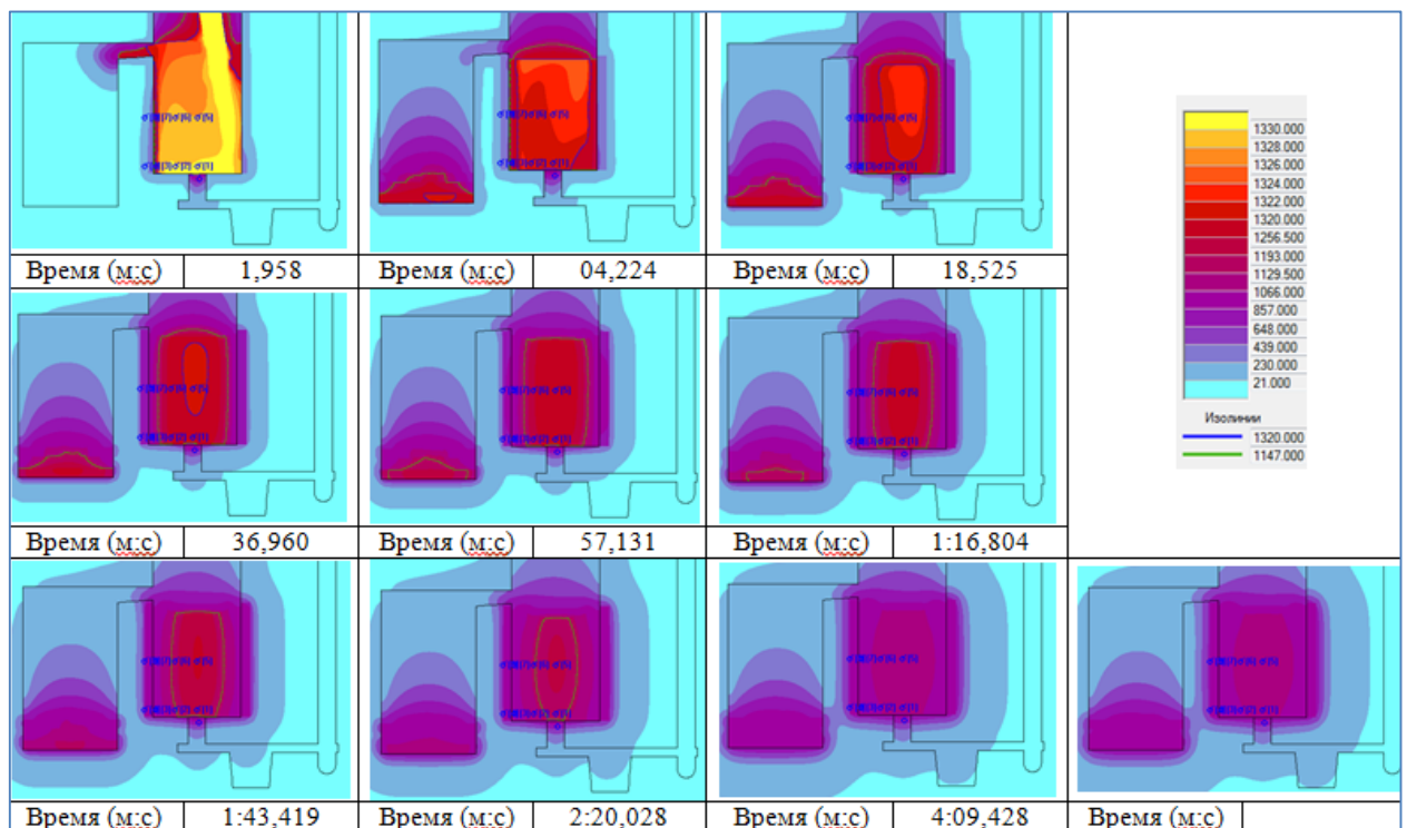
Рисунок 1 - Кинограмма распределения температур в объеме экспериментальной отливки «Цилиндр»
