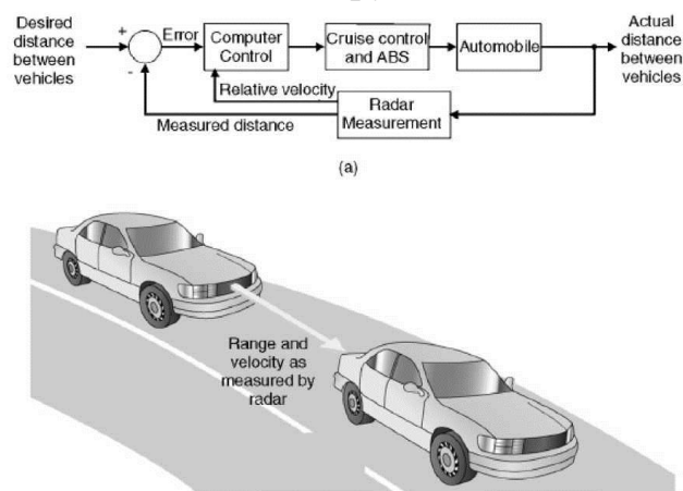
Рис. 3.2 Підсистема керування сучасним автомобілем – cruise control і ABS systems (Robert H. Bishop [1, 2])
