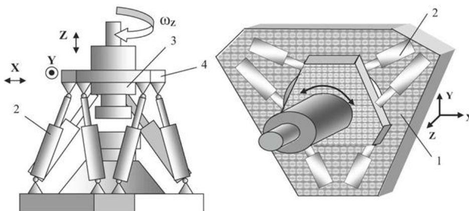
Рис. 9.3. Схема машини-гексапода
