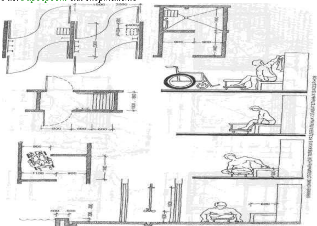
Рис. Гардеробні для спортсменів
