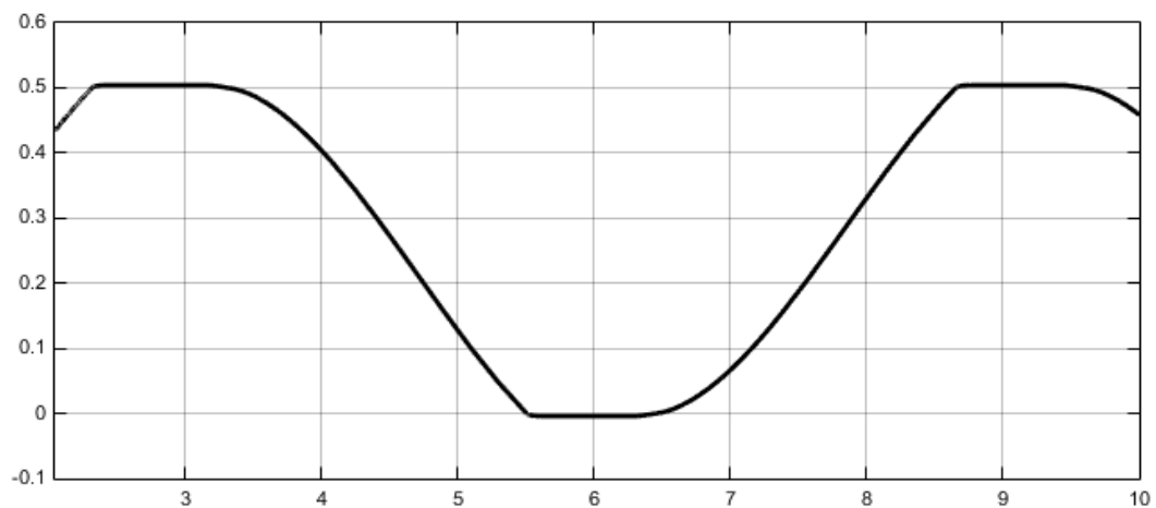
Рисунок Б.2 - Графік переміщення поршня гідроциліндру
