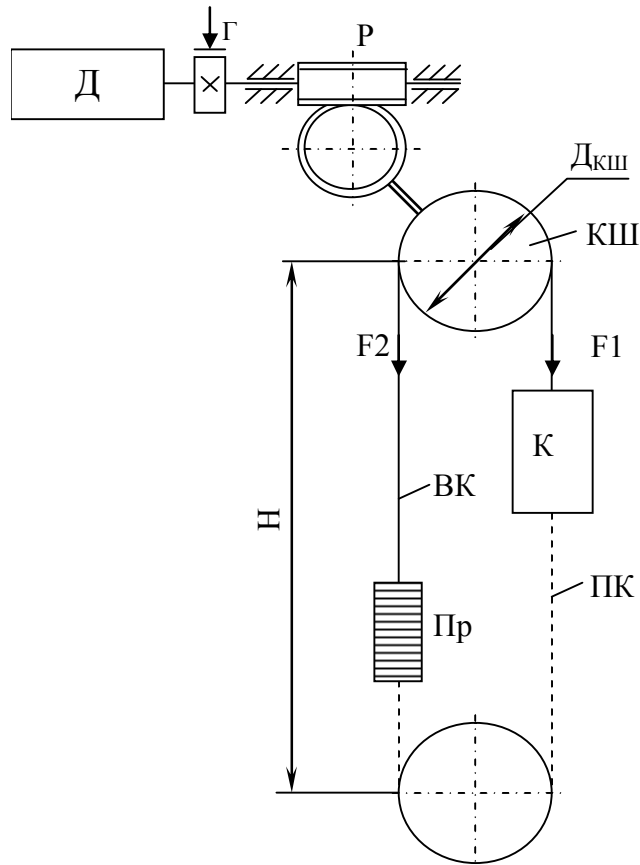
Д - двигун; Г - гальмо; Р - редуктор; КШ - канатоведучий шків; К - кабіна; Пр - противагу; ВК - врівноважує канат; ПК - підйомний канат
