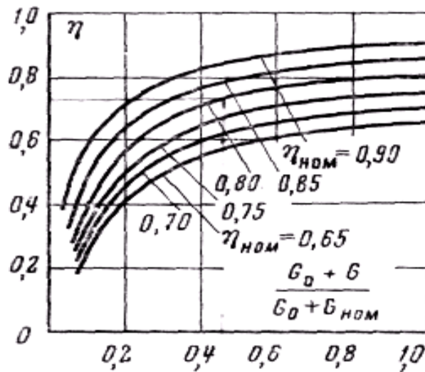
Рисунок 2 - Залежність \eta = f[(G_0 + G)/(G_0 + G_{nom})] при \eta = \text{const}
